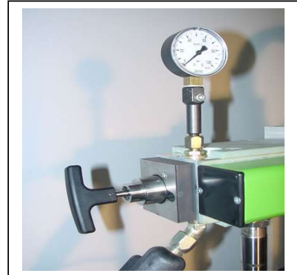
Bayonette-Filter an Traverse
