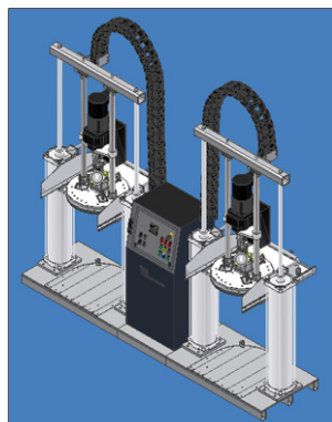
Tandem-Anlage mit automatischer Changeover-Funktion (optionale Ausstattung)
